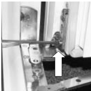
Anpressdruckverstellung mit Inbusschlüssel SW4.
